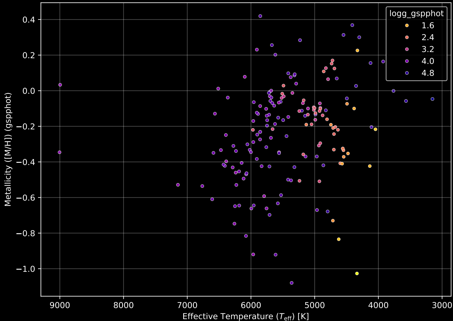
APOGEE DR17 Field: [288-28-O_TESS] Stellar Population Parameters (n= 170)
